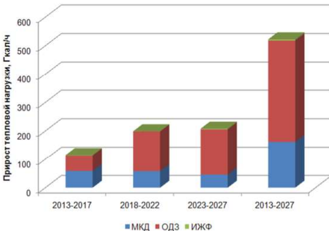
Рисунок 4.2 – Распределение прироста суммарной перспективной тепловой нагрузки по типам вводимых строений
