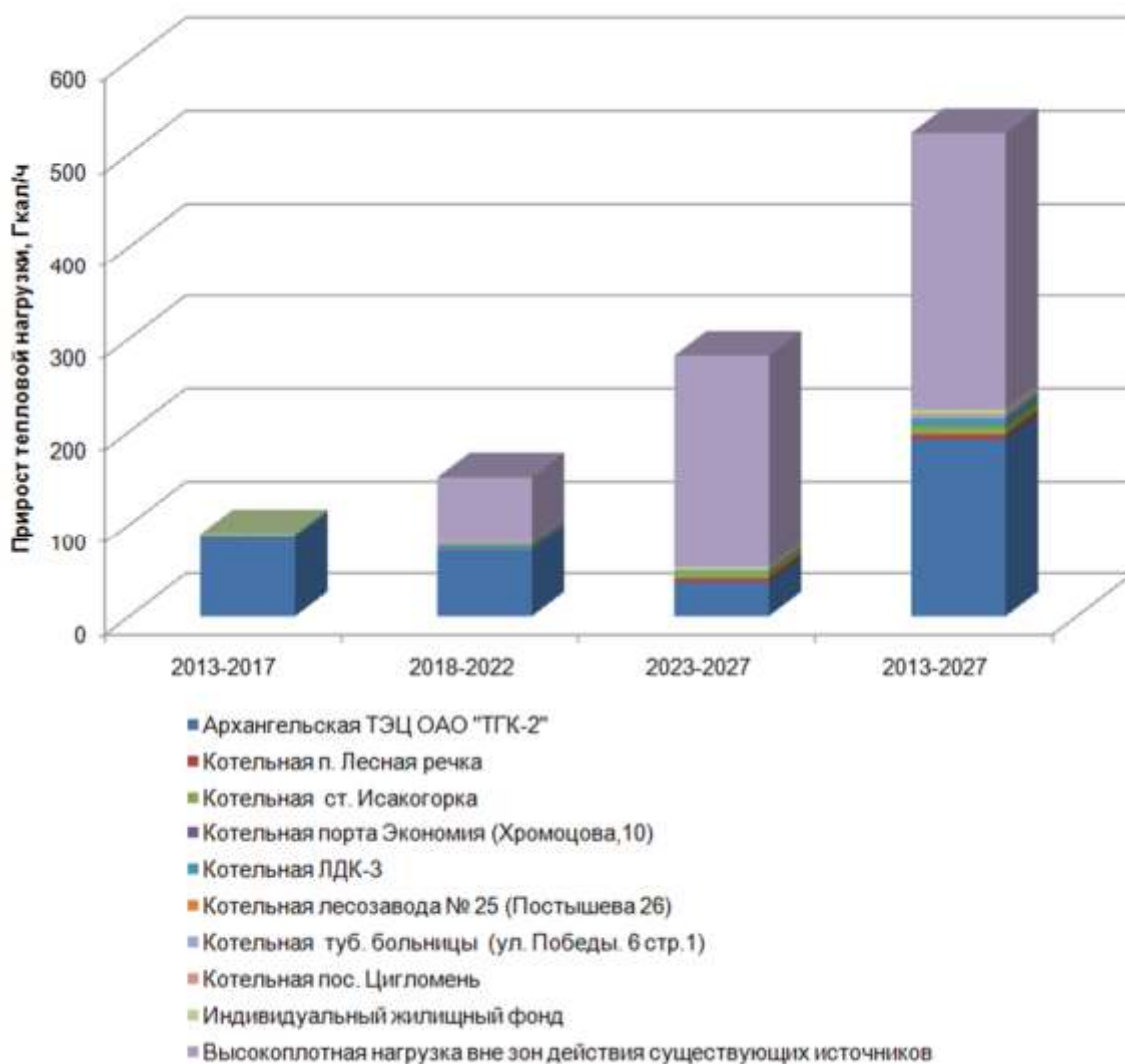
Рисунок 5.1 – Распределение прироста суммарной перспективной тепловой нагрузки по зонам действия источников
